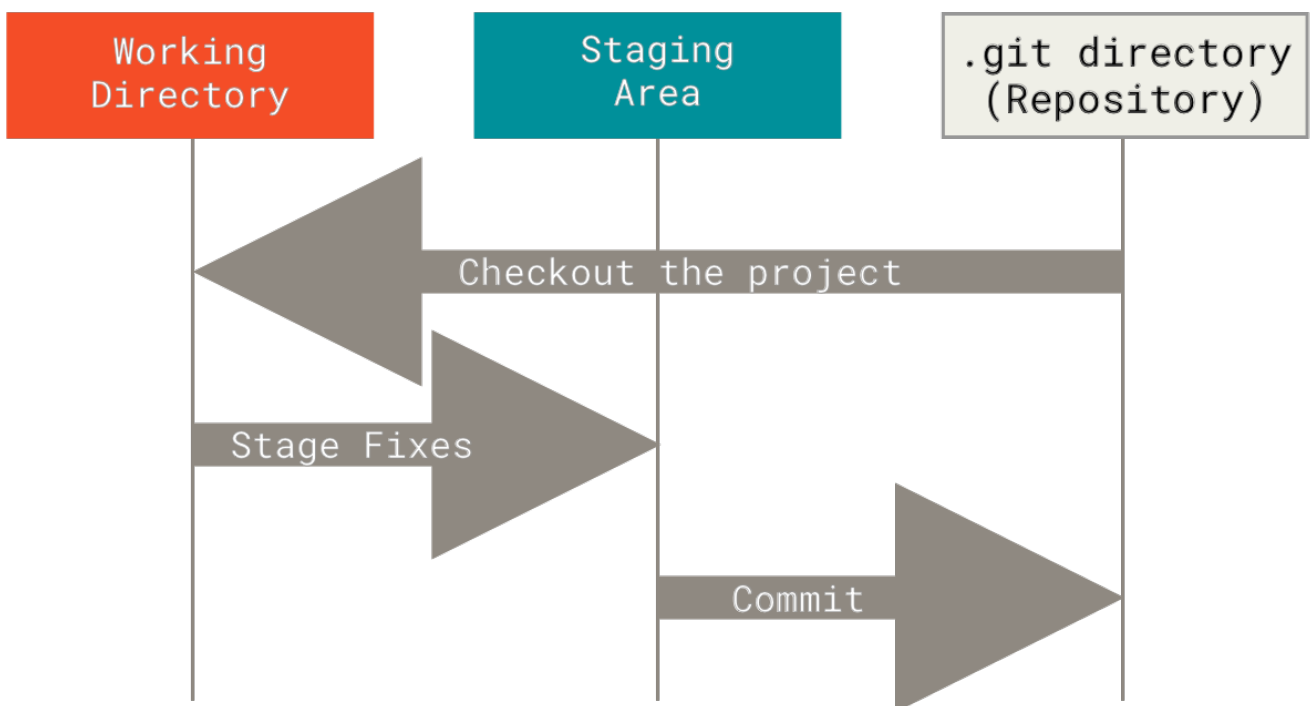
Рисунок 6. Рабочая директория, область подготовленных файлов и директория Git.
