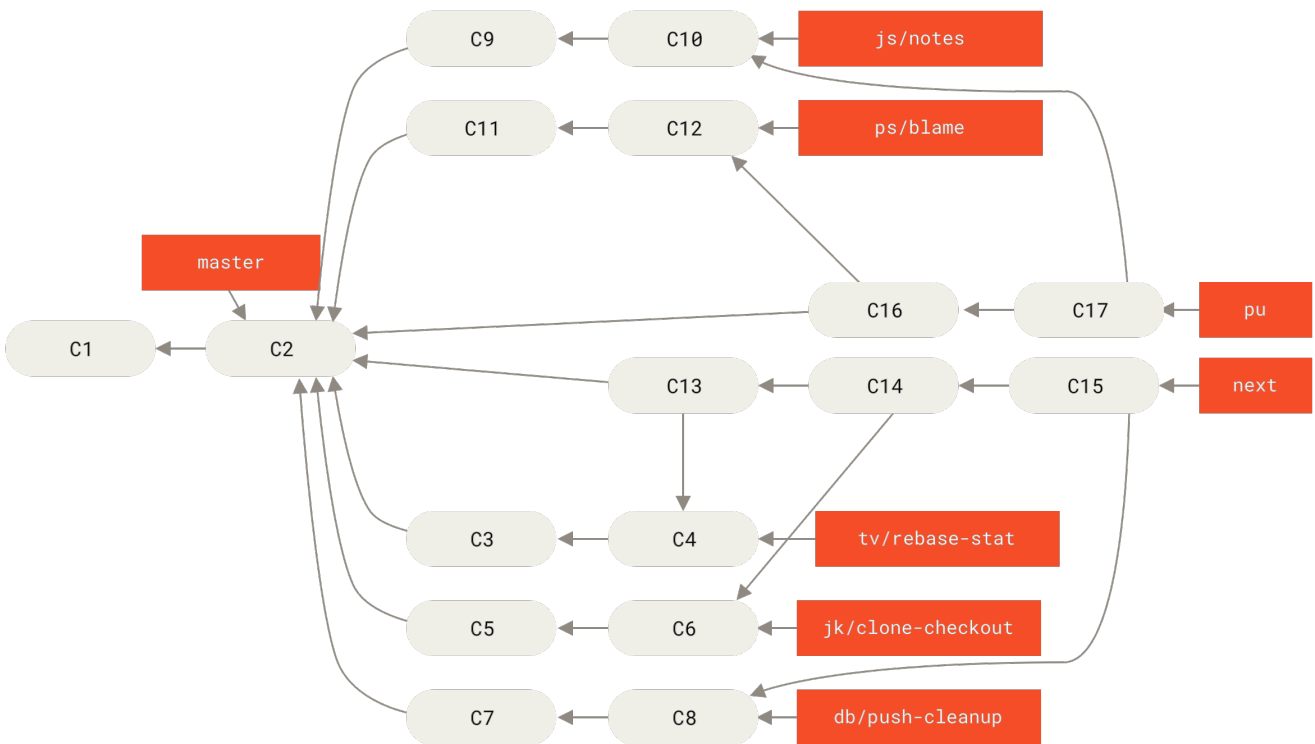
Рисунок 79. Слияние тематических веток в долгоживущие ветки интеграции.
